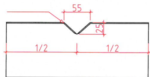
Griffausfräsung "V"
