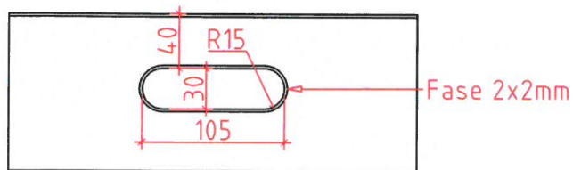
Griffausfräsung "O"
