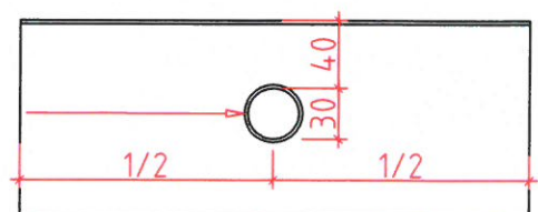
Griffausfräsung "K"
